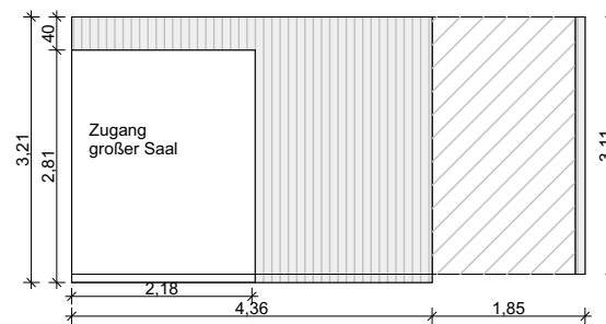
Innenansicht D
