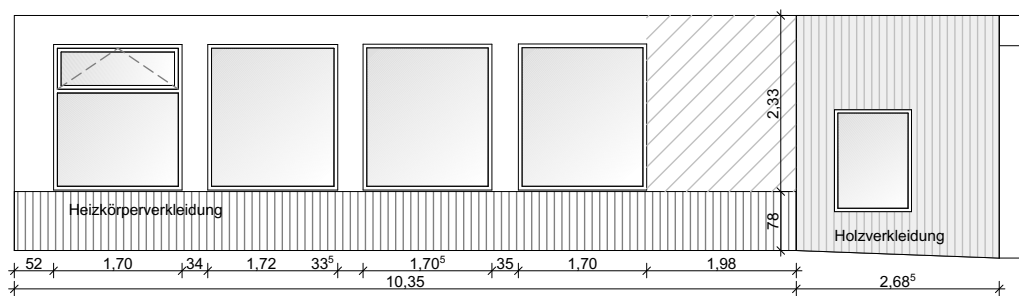
Innenansicht C
